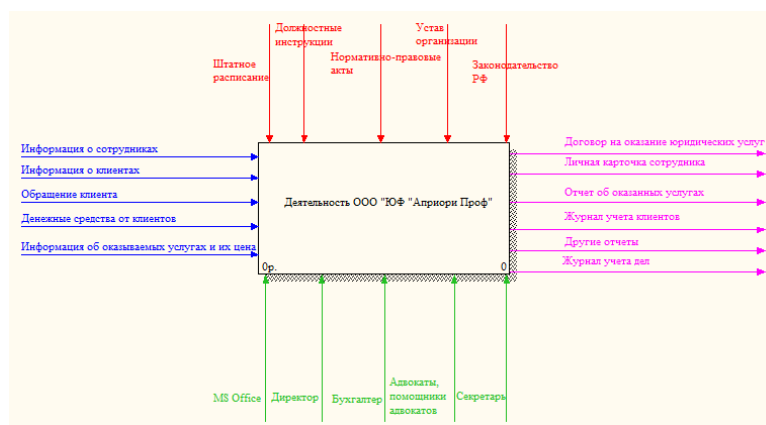
Рис. 1. Контекстная диаграмма IDEF0 AS-IS «Деятельность ООО «ЮФ «Априори Проф»»
