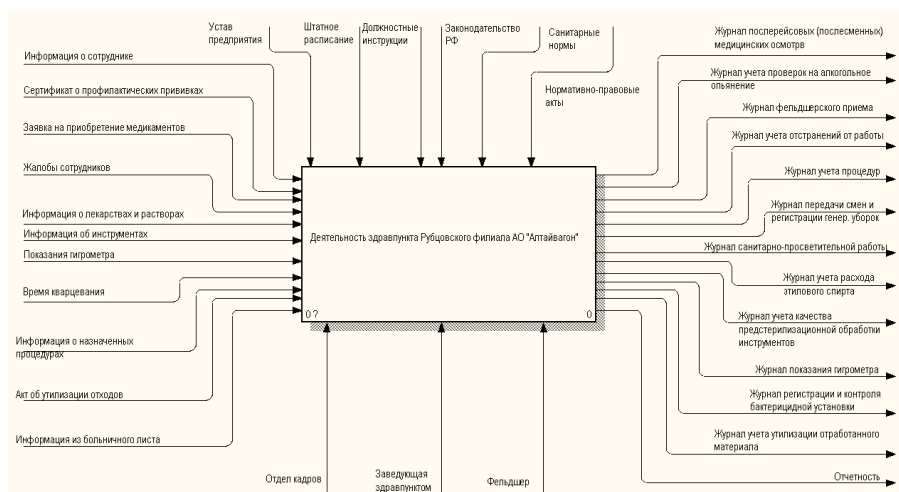
Рис. 1. Контекстная диаграмма IDEF0 AS-IS «Медицинская деятельность здравпункта Рубцовского филиала АО «Алтайвагон»»
